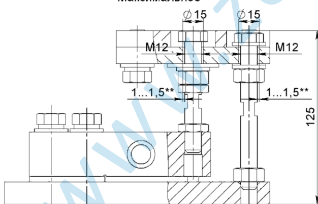
Свободно-опорное крепление датчика Максимальное
