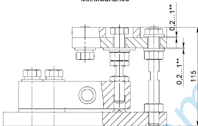
Свободно-опорное крепление датчика Минимальное
